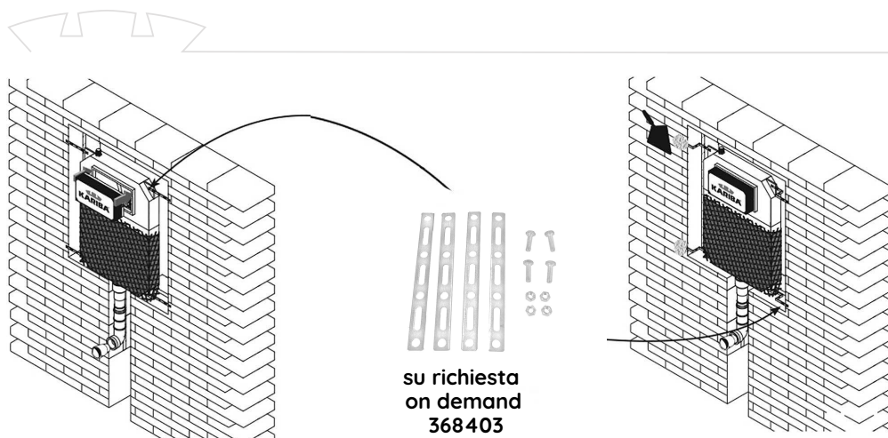
su richiesta on demand 368403 installazione Muratura Brick Wall
